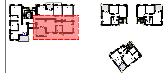
Planimetria generale
