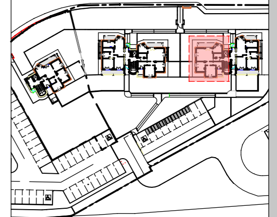
Planimetria generale
